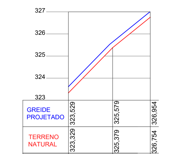
PERFIL LONGITUDINAL EIXO DA RUA JOSÉ LINS ESCALA H 1/1000 V 1/100
