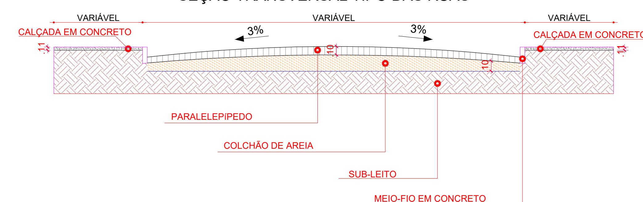
SEÇÃO TRANSVERSAL TIPO DAS RUAS
