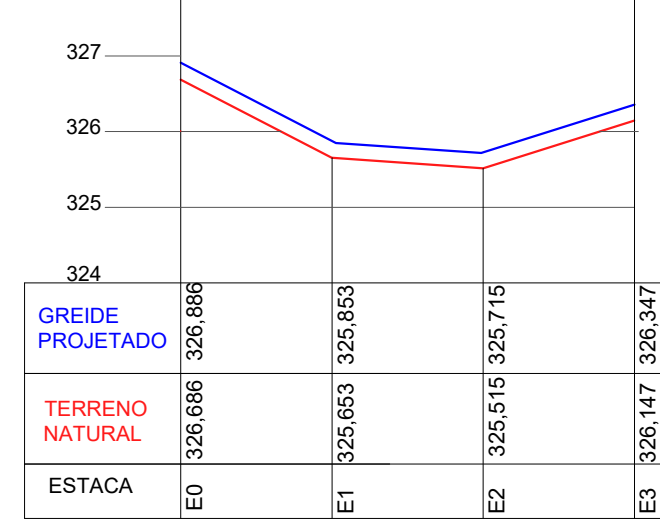
PERFIL LONGITUDINAL EIXO DA TRAVESSA 02 ESCALA H 1/1000 V 1/100
