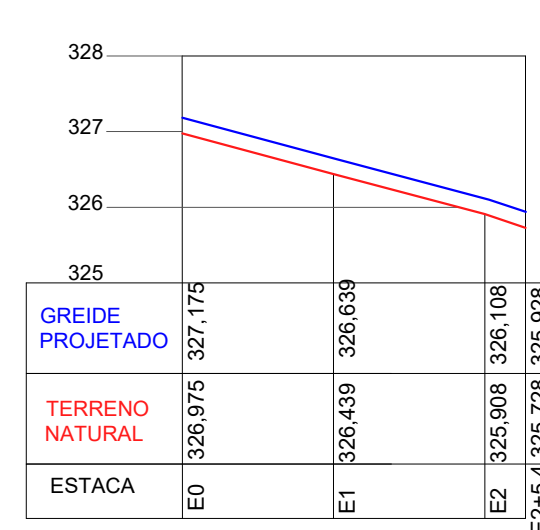
PERFIL LONGITUDINAL EIXO DA TRAVESSA 01 ESCALA H 1/1000 V 1/100
