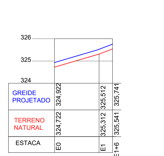
PERFIL LONGITUDINAL EIXO DA TRAVESSA 03 ESCALA H 1/1000 V 1/100
