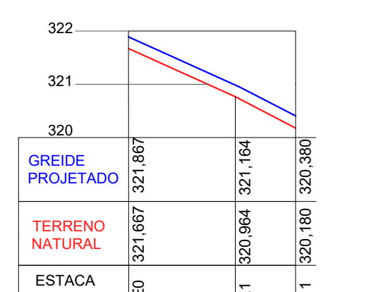
PERFIL LONGITUDINAL EIXO DA TRAVESSA 08 ESCALA H 1/1000 V 1/100
