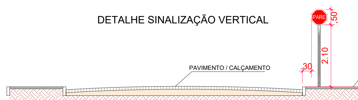
DETALHE SINALIZAÇÃO VERTICAL
