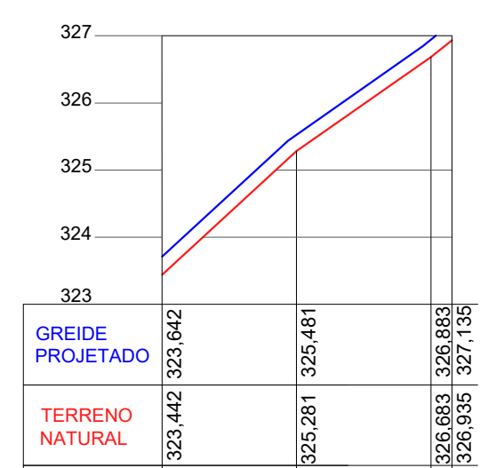
PERFIL LONGITUDINAL EIXO DA RUA JUSTINO CAVALCANTE ESCALA H 1/1000 V 1/100
