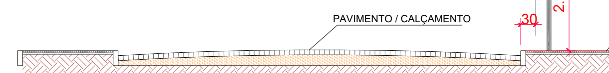
DETALHE SINALIZAÇÃO INDICATIVA DE RUAS
