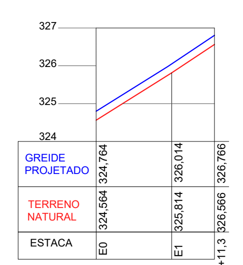
PERFIL LONGITUDINAL EIXO DA TRAVESSA 07 ESCALA H 1/1000 V 1/100
